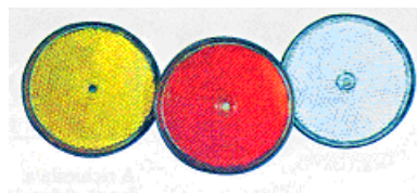
Catarifrangente Ø 80 con foro Arancio – Cod. R004.02.10A Bianco – Cod. R004.02.23A Rosso – Cod. R004.02.24A
